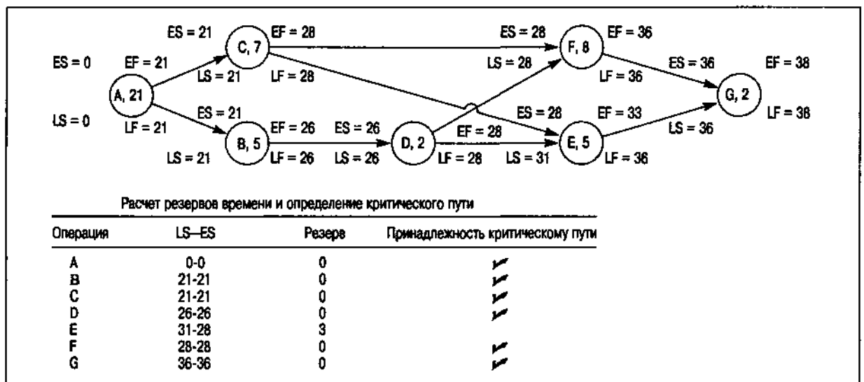
Рис. 3.4. Расчет параметров сетевого графика проекта создания новой модели компьютера
