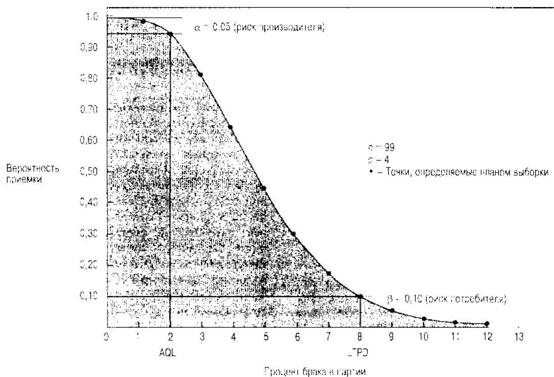
Рис. 6д.1. Оперативная характеристика для AQL = 0,02, α = 0,05; LTPD = 0,08 и β = 0,10
