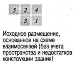
Рис. 10.9. Решение задачи о размещении пяти отделов в магазине методом системной планировки
