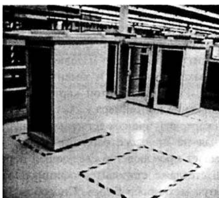
Рис. 8.5. Пополнение запасов деталей с помощью сигнального маркера
