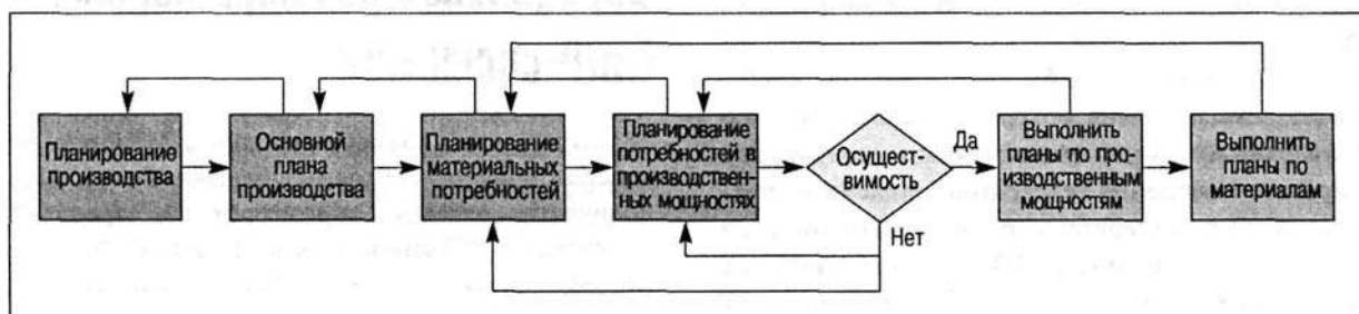
Рис. 16.10. MRP-система с замкнутым циклом (на схеме показаны петли обратной связи)
