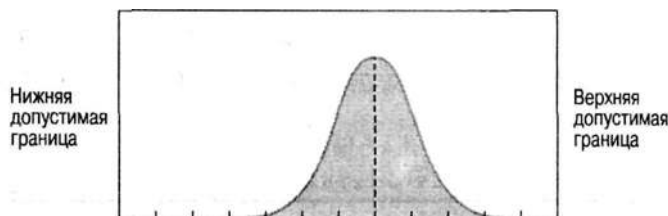
Рис. 6д.4. Производственные возможности процесса
