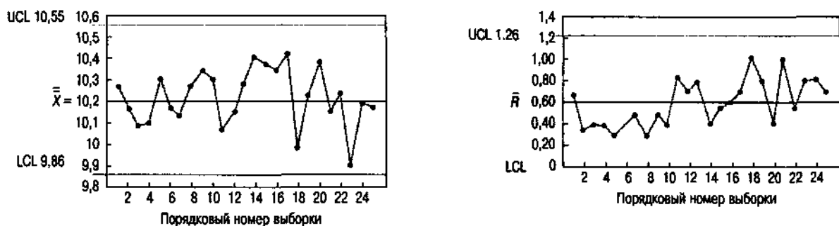
Рис. 6д.3. Карты типов X и R для примера 6д.3
