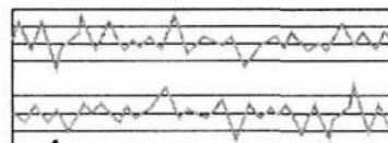
График временной последовательности, отображающий статистические значения с указанием среднего значения и одного или нескольких контрольных пределов, определенных статистически
